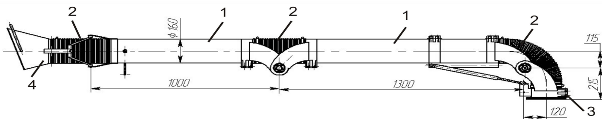
Рис. 3 Схема РВУ-3/160
