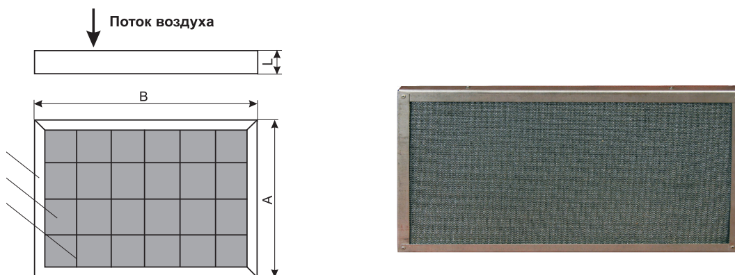
Рис.1 Схема фильтра ФяЖ.
