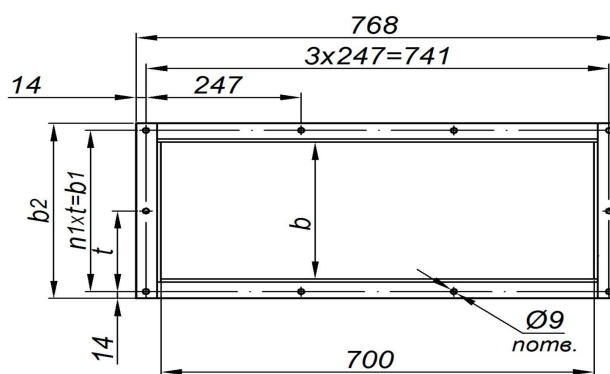
Рис. 13 Фланец входа грязного воздуха фильтров ФПИ-4; ФПИ-8; ФПИ-12 и ФПИ-16.
