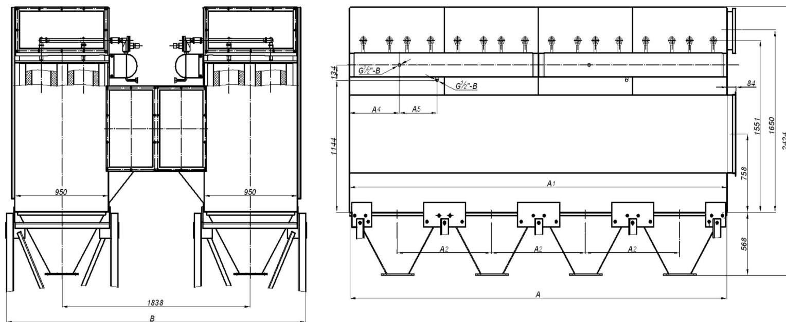
Рис.11 Схема фильтра ФПИ-32.
