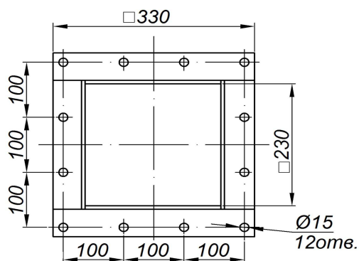
Рис. 14 Фланец бункера фильтров ФПИ-4; ФПИ-8; ФПИ-12 и ФПИ-16.
