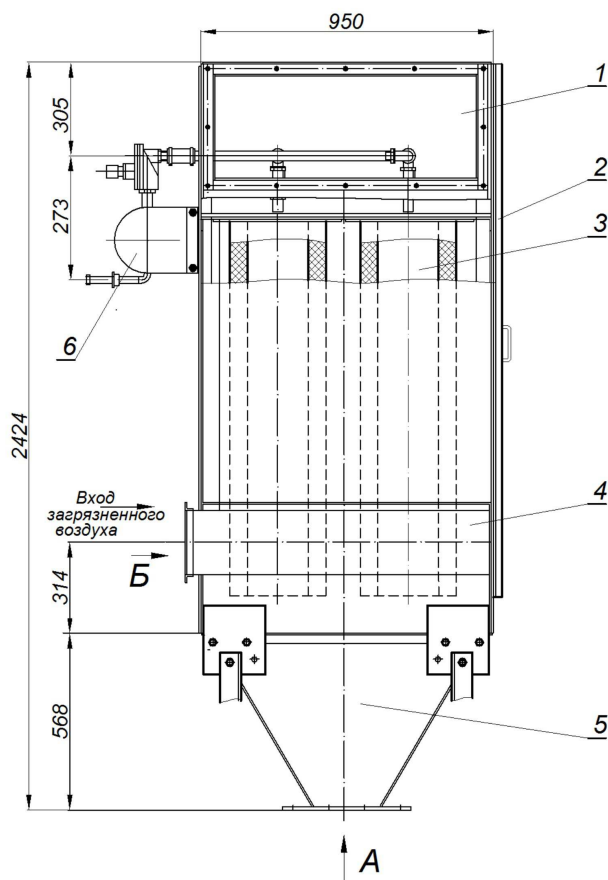
Рис.2 Схема фильтра ФПИ-2
