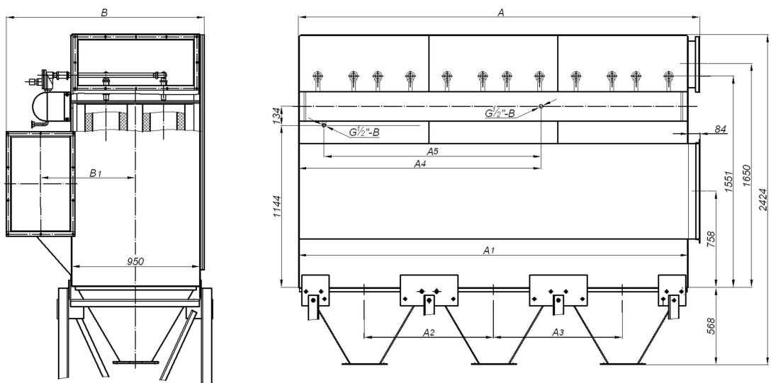
Рис. 8 Схема фильтра ФПИ-10; ФПИ-12
