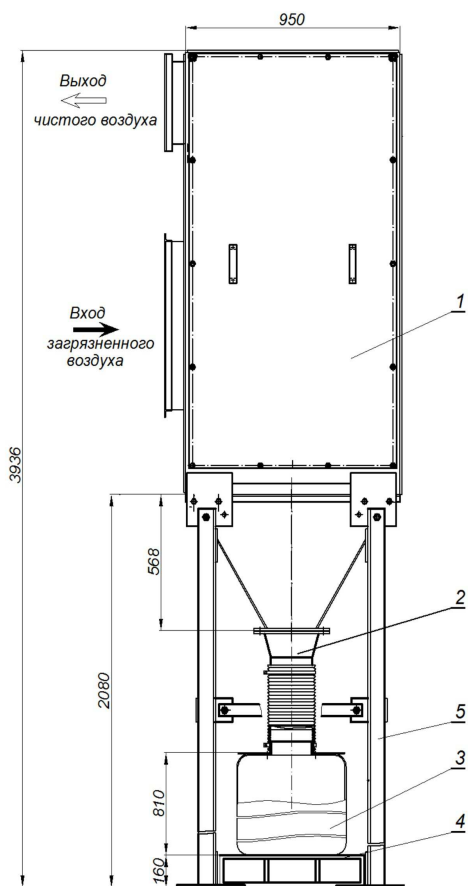
Рис.1 Схема фильтра ФПИ-4 со стандартными опорами
