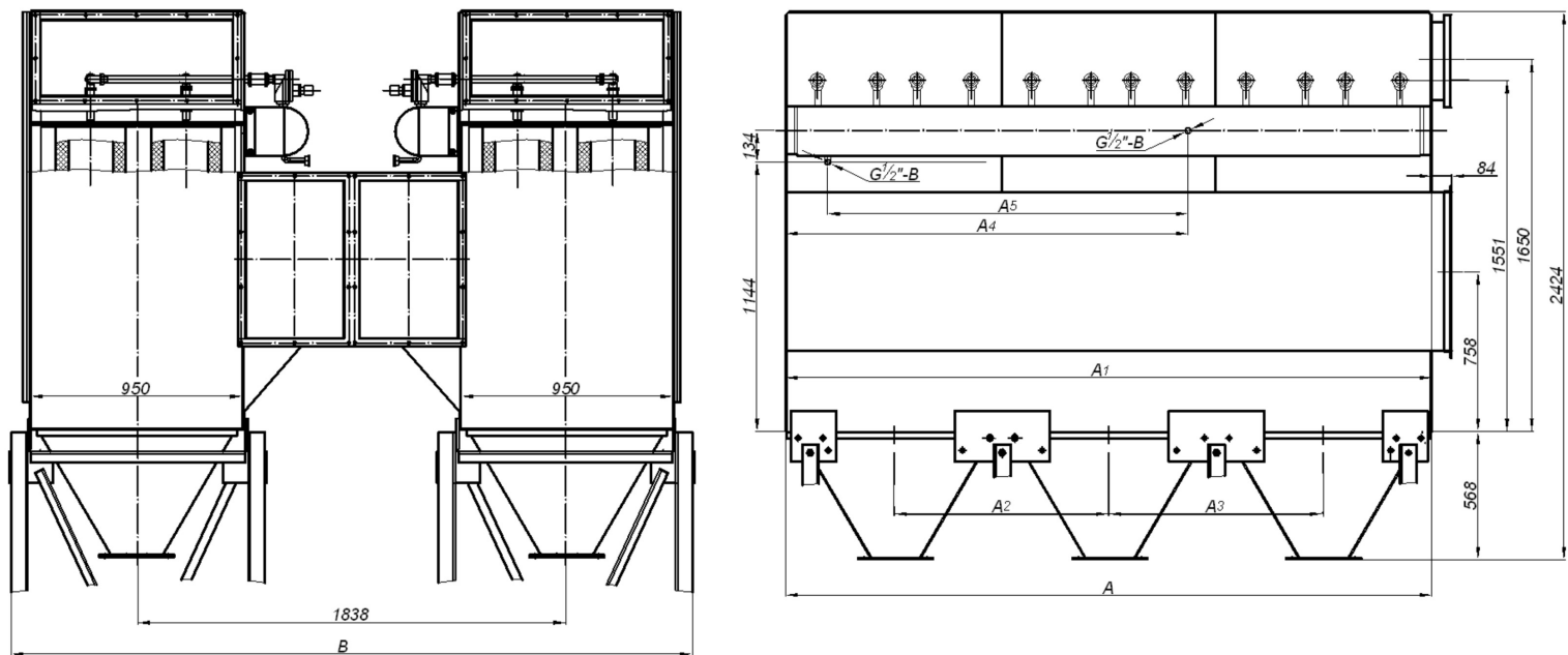
Рис.10 Схема фильтра ФПИ-20; ФПИ-24.
