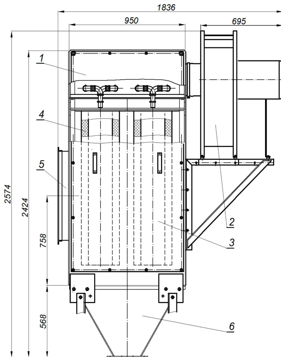
Рис. 5 Схема фильтра ФПИ-4А
