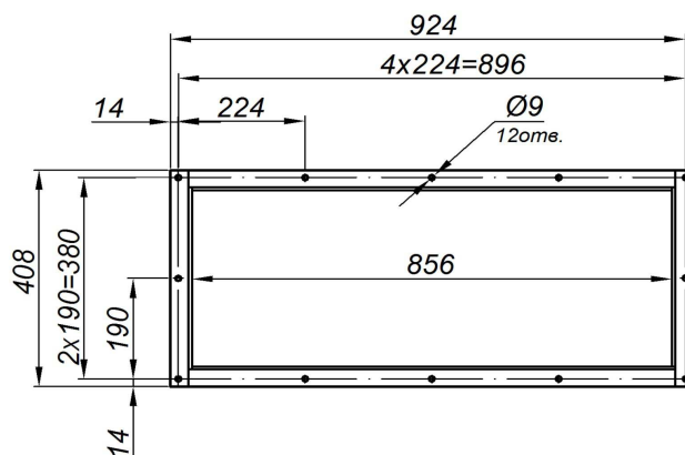
Рис. 12 Фланец выхода чистого воздуха фильтров ФПИ-4; ФПИ-8; ФПИ-12 и ФПИ-16.
