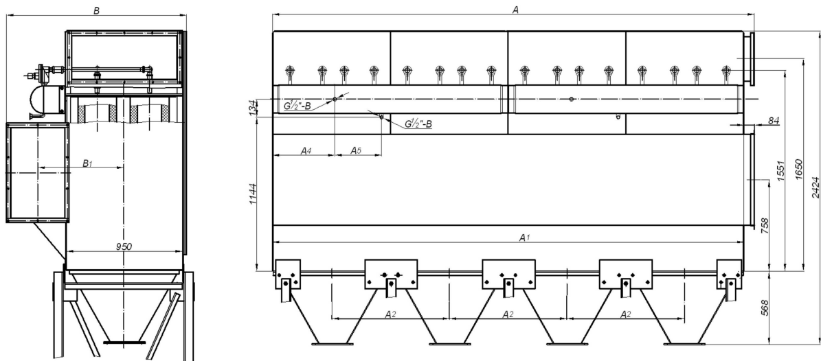
Рис. 9 Схема фильтра ФПИ-16.
