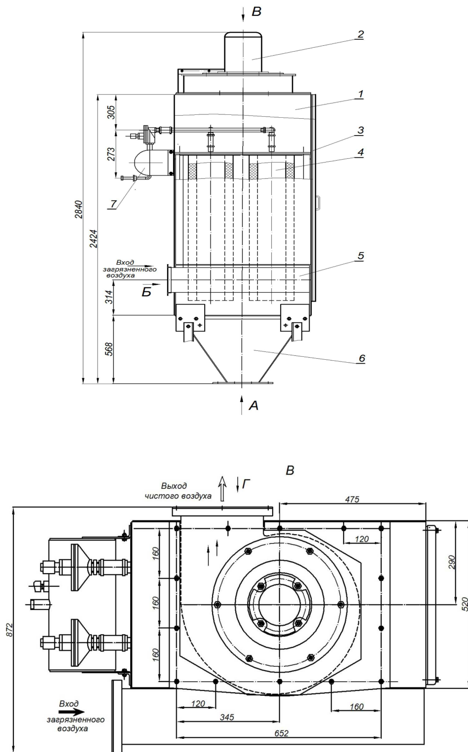
Рис.4 Схема фильтра ФПИ-2А
