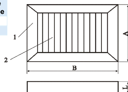
Рис.1 Схема фильтра ФяС-Ф-ПМП.
