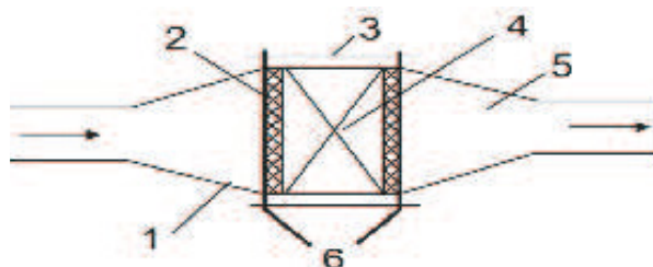
Рис.5 Схема одиночной установки фильтров ФяС в воздуховоде.
