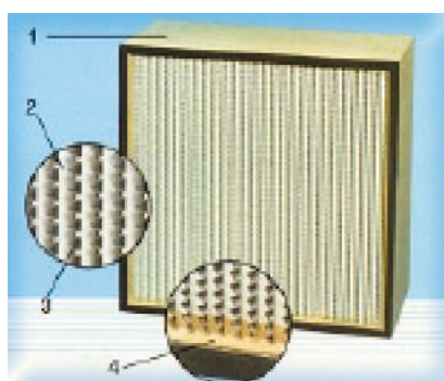
Рис.1 Фильтр с алюминиевыми сепараторами 1- корпус; 2- фильтрующий материал; 3- сапараторы из алюминиевой фольги 4- специальный герметик;;
